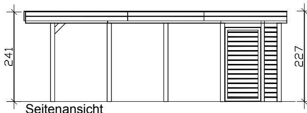
Seitenansicht
