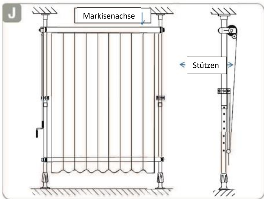
Vorderansicht
