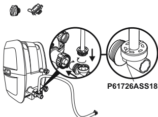
Kicsavarozható felfújó/leeresztő szelep
