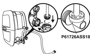
Schnellventil zum Aufblasen und Entleeren
