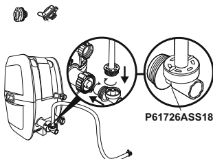
Válvula de enchimento/ esvaziamento rápido
