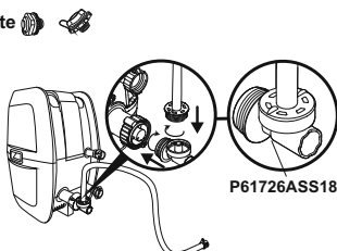
Valvola di gonfiaggio/ sgonfiaggio rapido
