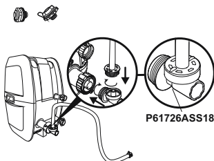
Válvula de inflado/ desinflado rápido
