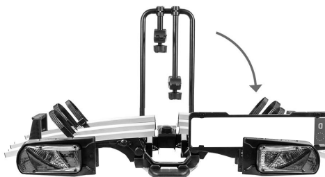
Figure 9 : Étape 2
