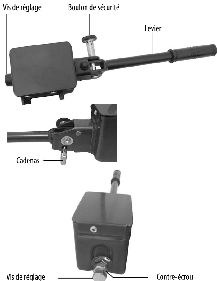
Figure 7 : Fermeture rapide
