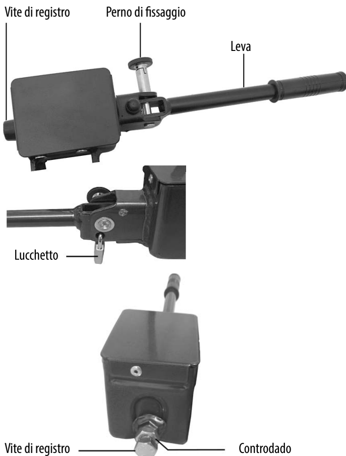
Figura 7: Aggancio rapido
