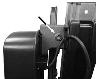
Bild 2: Montage Rückleuchten
