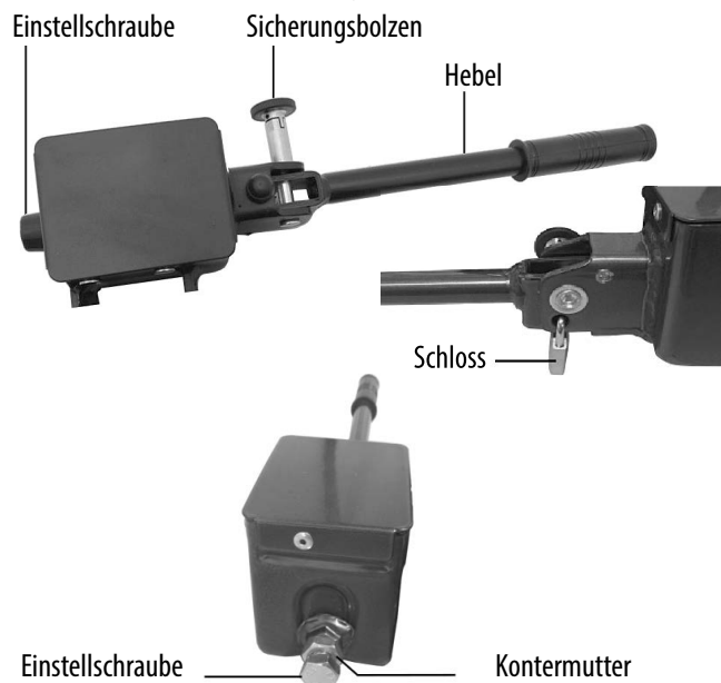
Bild 7: Schnellverschluss
