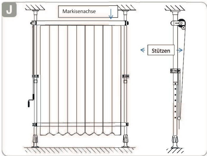
Vorderansicht
