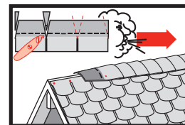
Verschneiden der Schindelungen für First
