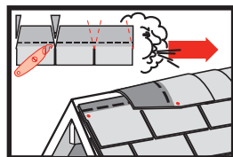
Coupez les jupes comme illustré pour les faitièrès
