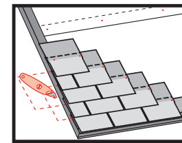
Snij de tabs zoals getoond voor correcte verlegging
