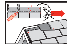
Snij de tabs zoals getoond voor nokafdekking
