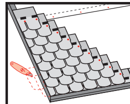
Schindelungen abschneiden wie angedeutet
