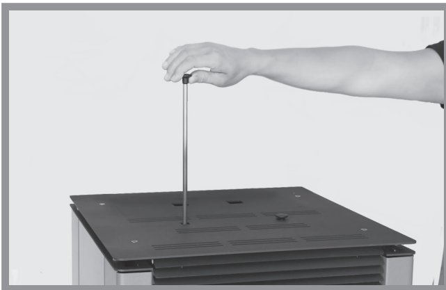
Abb. 12e: Reinigung der Wärmetauscher
