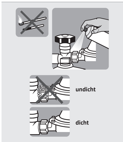
Abb.2: Dichtheitsprüfung
