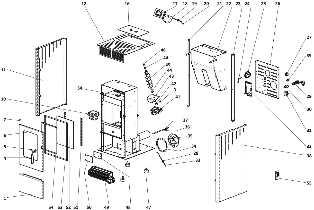
Abb. 14 Explosionszeichnung
