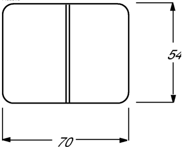
Maßbild
