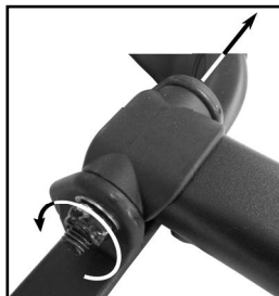
Bild 2: Gelenkschraube entfernen
