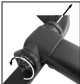
Fig. 2 : retirer la vis d'articulation
