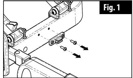
Bild 3: Entfernen der Halteklammern
