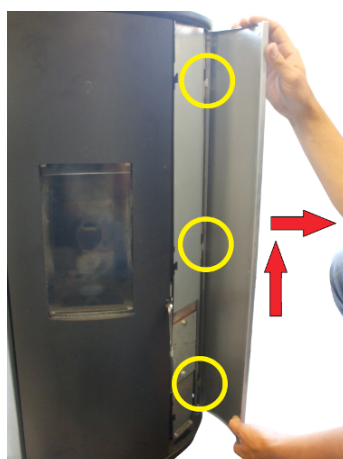
Fig. 66 - Sfera 3 / Sfera 3 Plus: Die Seitenplatten auslösen
