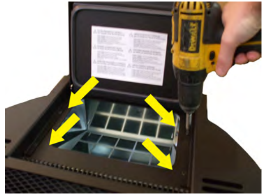
Fig. 68 - Lösen der Schrauben des Deckels 2
