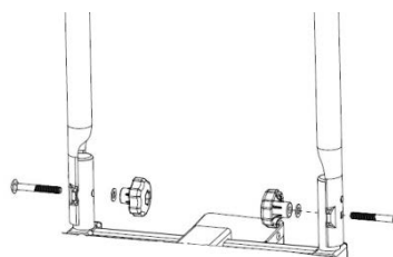
Obrázek 2: Montážní U-konzola
