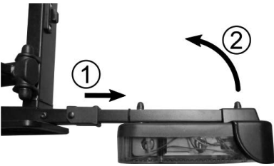
Figura 18: Ripiegamento fanale posteriore
