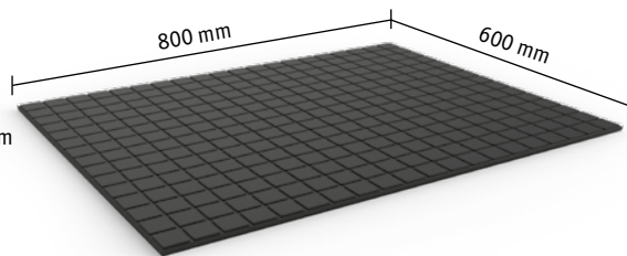
Ansicht Plattenoberseite
