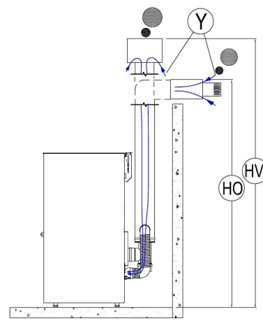
Fig. 12 - Anschlüsse Rauchabzugsrohr
