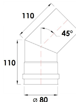
Fig. 21 - Krümmer 45°
