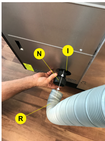
Fig. 10 - Flexibler Schlauch
