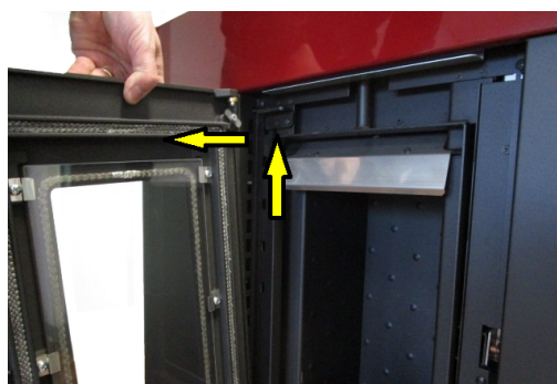
Fig. 28 - Ausbau der Tür
