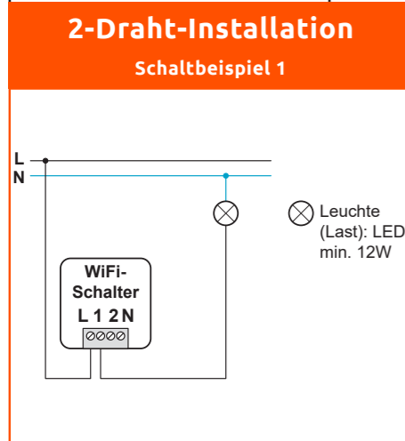
WiFi-Wechselschalter als Ausschalter
