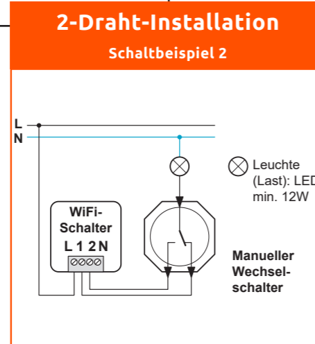
WiFi-Wechselschalter mit einem zusätzlichen manuellen Wechselschalter
