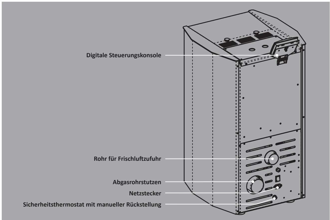
Abb. 1a: Geräteübersicht (Abbildung modellabhängig)
