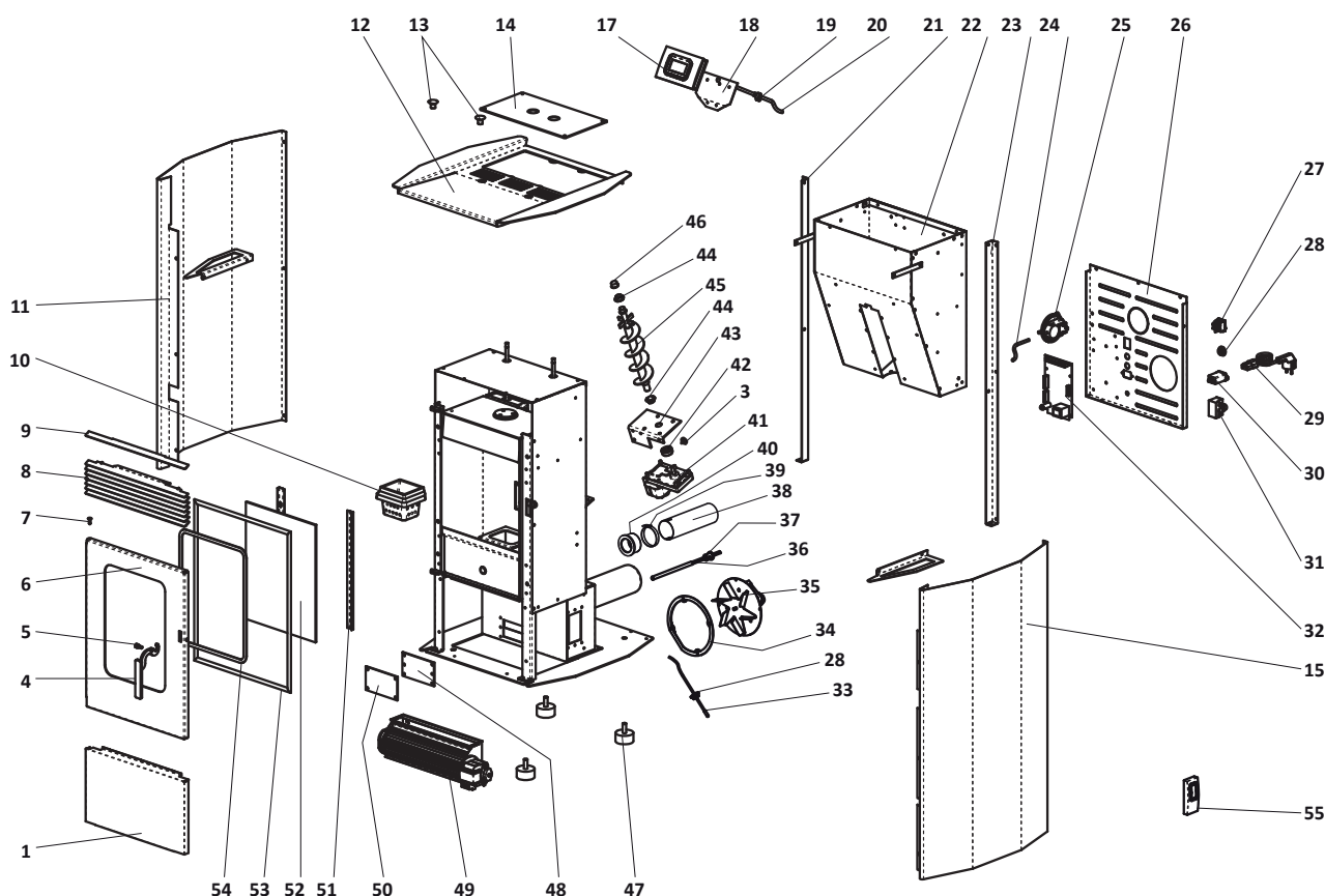
Abb. 14 Explosionszeichnung
