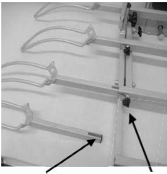
Warnmarkierung Knaufschraube
