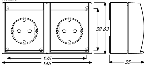
Maßbild
