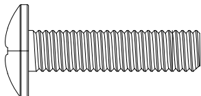
C Rundkopfschraube / vis à tête ronde ronde kopschroef / M6*25 (x14)
