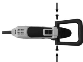
Bild 9: Schutzkappe festschrauben
