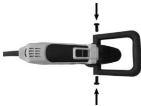
Afb. 9: Beschermkap vastschroeven
