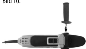
Bild 11: Zusatzhandgriff montieren
