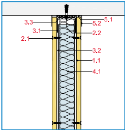
Anschluss an Massivdecke
