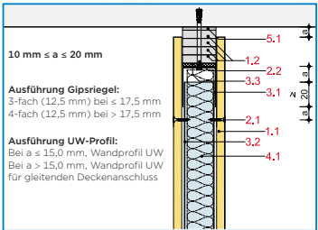
Gleitender Anschluss an Massivdecke
