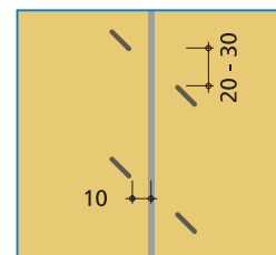
Versetzte Verklammerung
