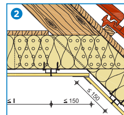
Anschluss der Dachschräge an Kehlbalkendecke mit dem flexiblen Rigips AquaBead Flex PRO
