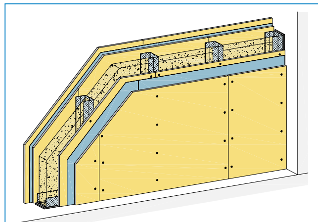
Metall-Einfachständerwand 3-lagig beplankt gem. Widerstandsklasse RC2
