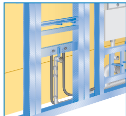
Einbau eines Waschbecken- ständers für einfache Wasch- becken
