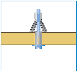
Hohlwanddübel, z. B. Molly-Schraubanker, Hilti HDD)
