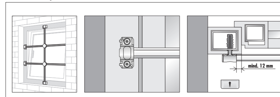
Abb. 1: Rahmenmontage
