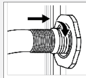
4. Um das Ventil nun zu öffnen und den Wasserfluss zu ermöglichen, drehen Sie den Anschluss im Uhrzeigersinn, während Sie den Anschluss zur Spa bewegen, bis dieser schließlich einrastet.
