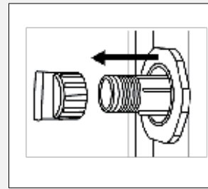
2. Herausgezogene, geschlossene Position. Ziehen Sie das Ventil bis zum Anschlag heraus. Entfernen Sie nun den Deckel.
