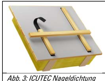
Abb. 3: ICUTEC Nageldichtung
